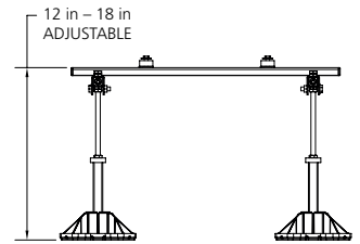
Mini Frame BN8100 & Extension Kit BN8101
